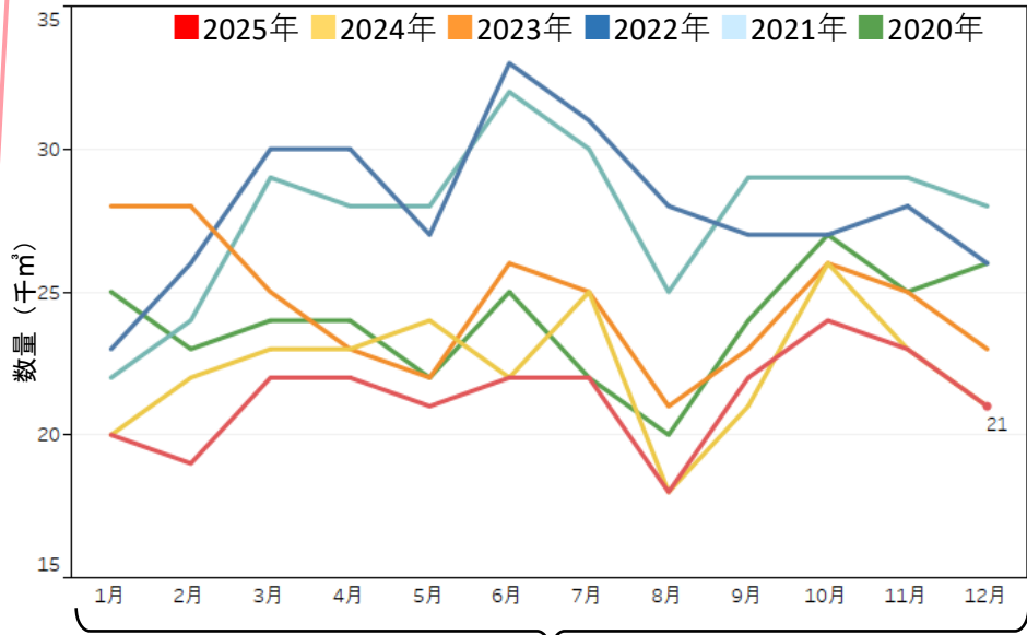
製材品出荷量の月別推移 (中部地区)
